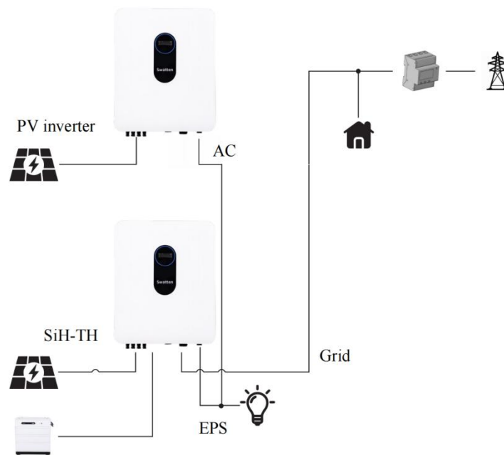
Abbildung 2-6 EPS-Terminal zur Nachrüstung der bestehenden PV-Anlage
